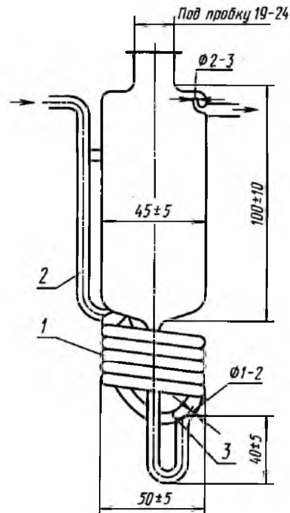
1 — пять полных витков трубки диаметром (6 \pm 1) мм; 2 — стеклянная перемычка; 3 — место впаива газопроводящей линии
